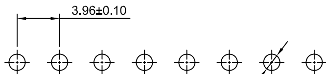
P.C.B LAYOUT
